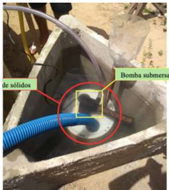
Figura 14. Filtro de sólidos e bomba submersa instalados adequadamente dentro do sedimentador (Fonte: acervo pessoal do autor).
